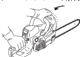
チェーンブレーキ解除
