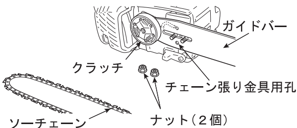
ソーチェーンの向き
